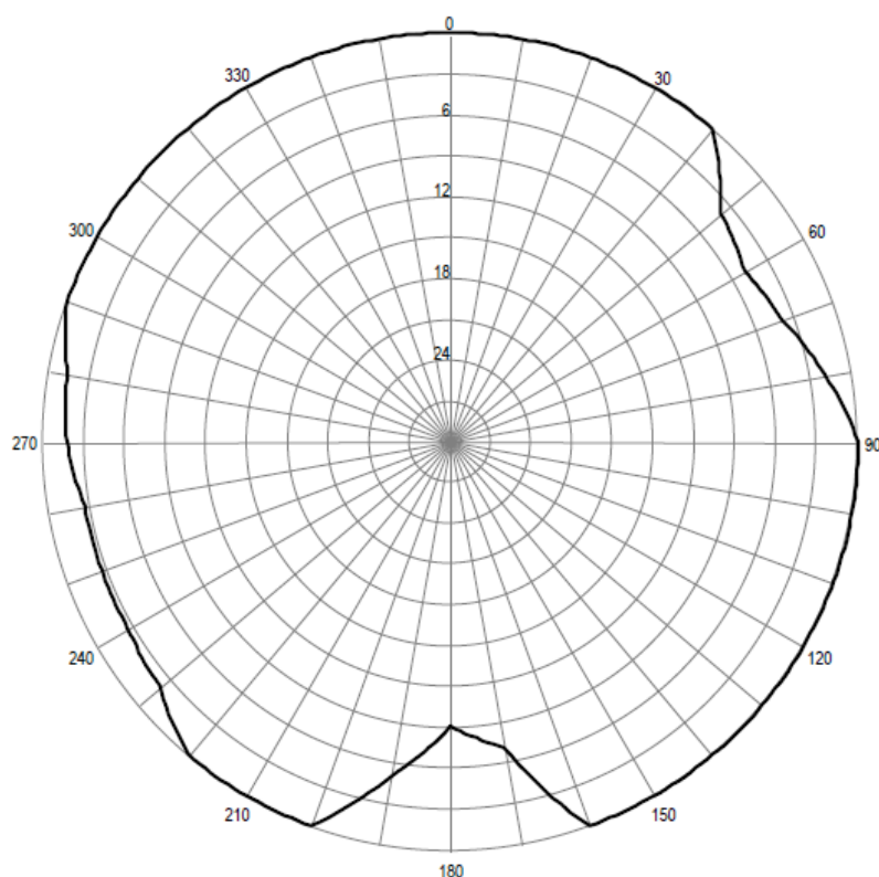
Pozioma charakterystyka promieniowania anteny stacji Suwałki 93,10 MHz
