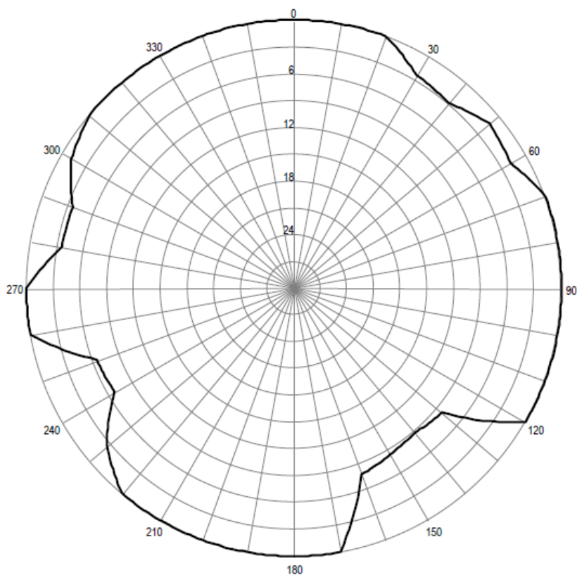
Pozioma charakterystyka promieniowania anteny stacji Elk 90,70 MHz
